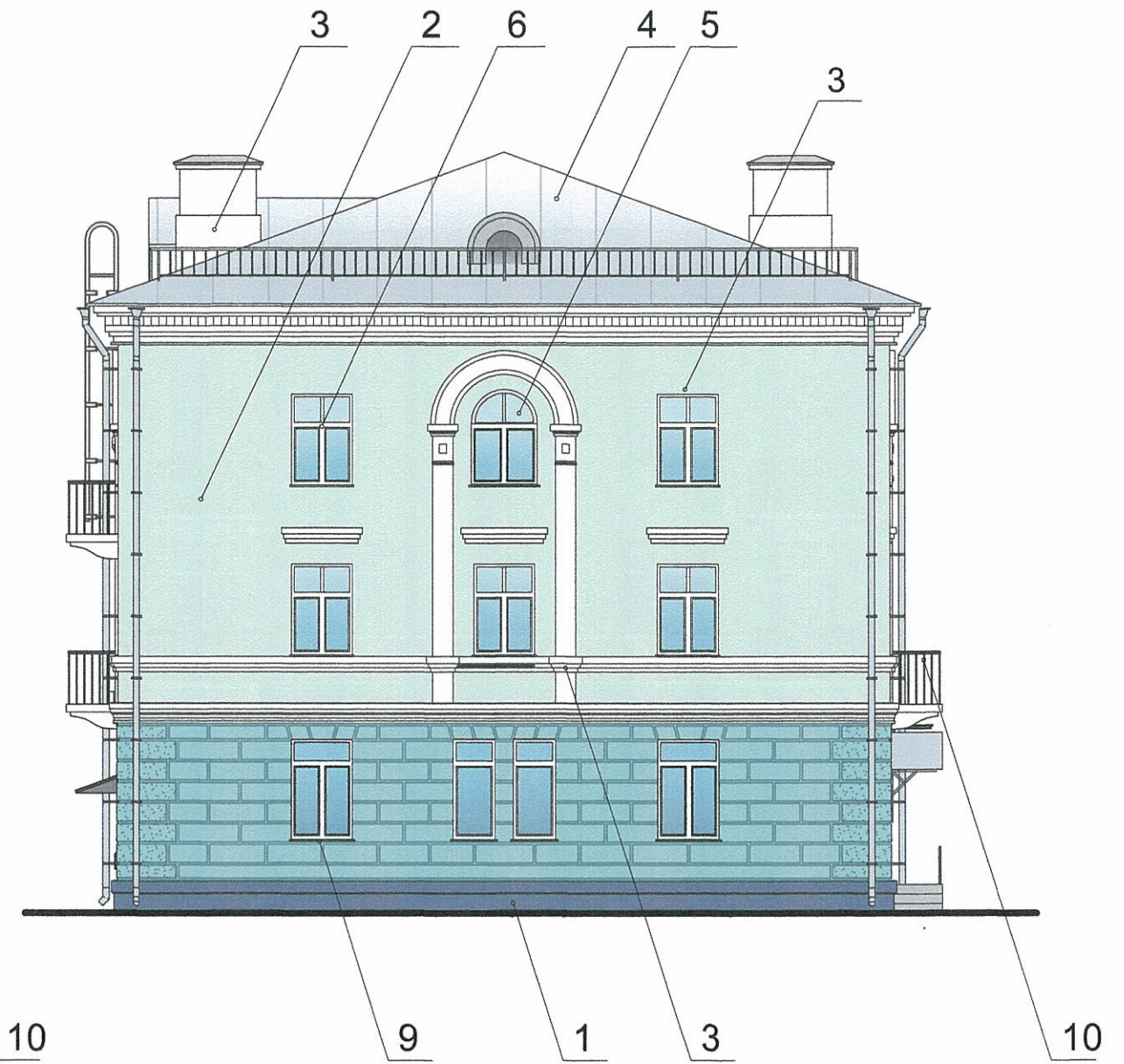
Торцевой фасад
