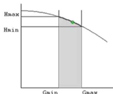
Рисунок 16 – Напорно-расходная характеристика насоса
