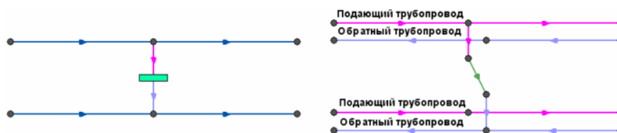
Рисунок 2.28. Слева: однолинейное изображение сети, справа: её внутреннее представление
