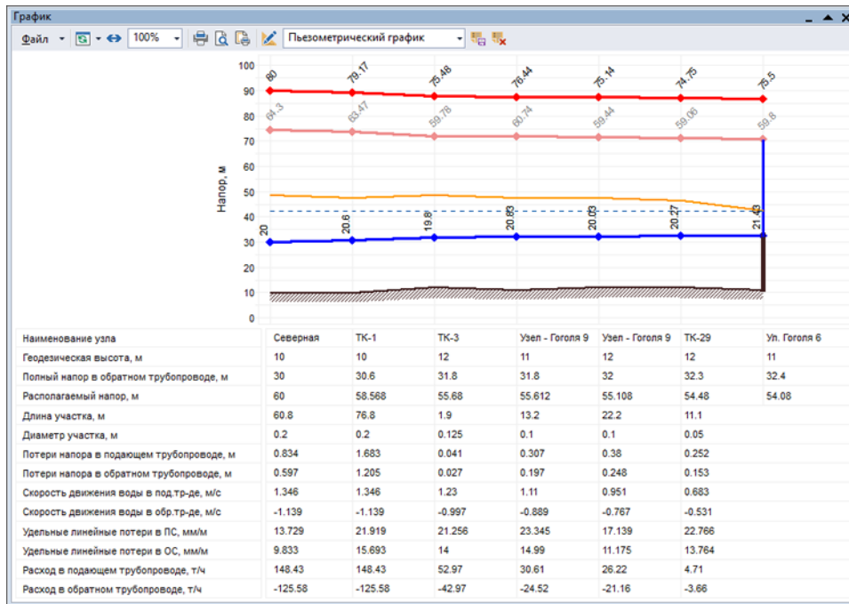
Рисунок 17.8. Совмещение пьезометрических графиков
