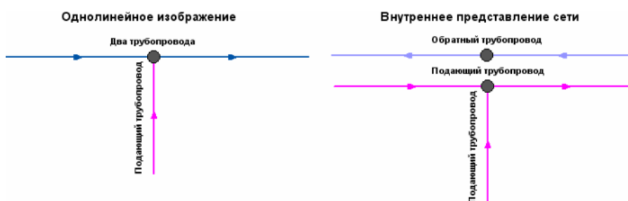
Рисунок 2.13. Подключение подающего трубопровода к тепловой сети
