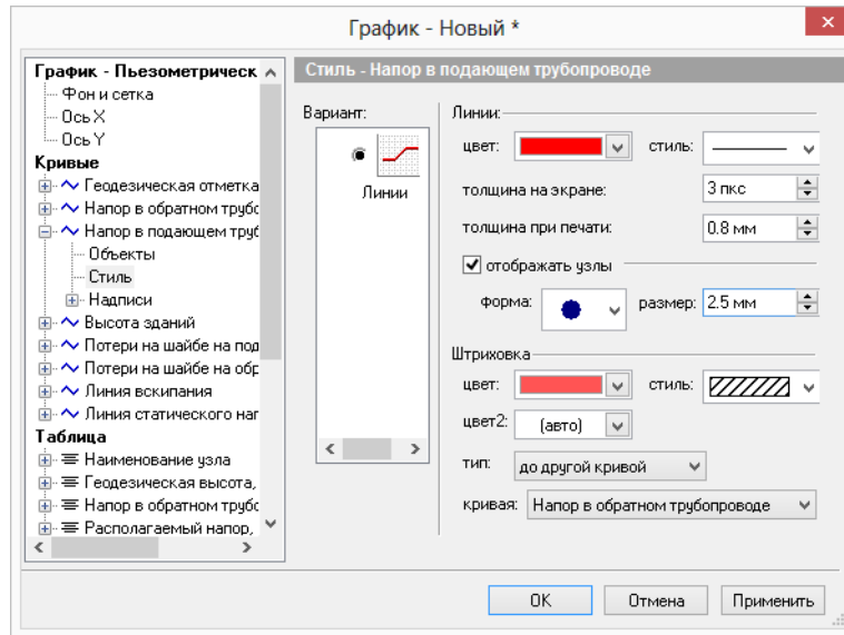
Рисунок 17.22. Настройка штриховки
