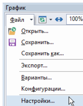
Рисунок 17.33. Настройки графика
