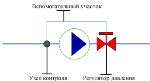
Рисунок 2.38. Регулятор давления «до себя» на подающем трубопроводе
