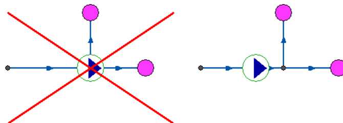
Рисунок 2.19. Слева: неправильное изображение насоса, справа – правильное
