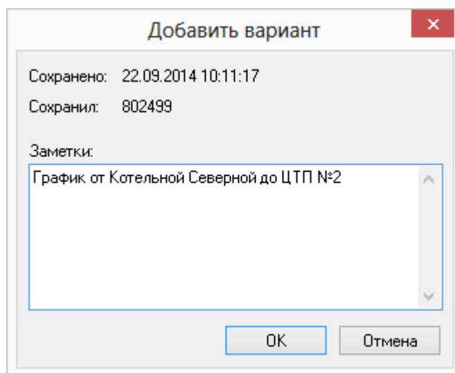
Рисунок 17.5. Варианты графика
