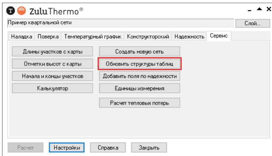
Рисунок 25.2. Обновление таблиц
