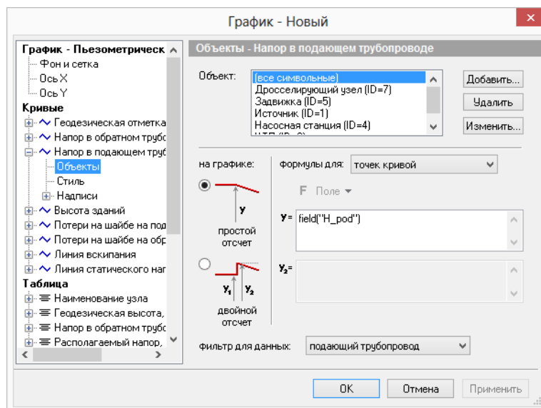
Рисунок 17.19. Подраздел «Объекты»
