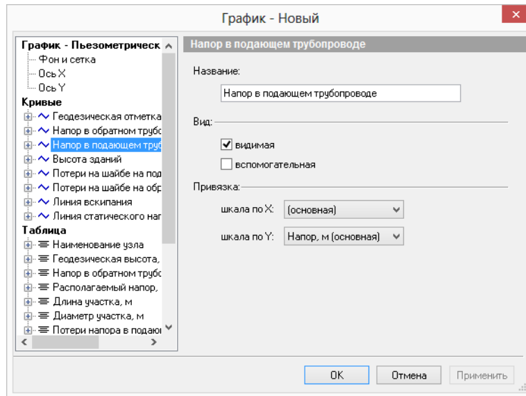
Рисунок 17.18. Настройка кривой
