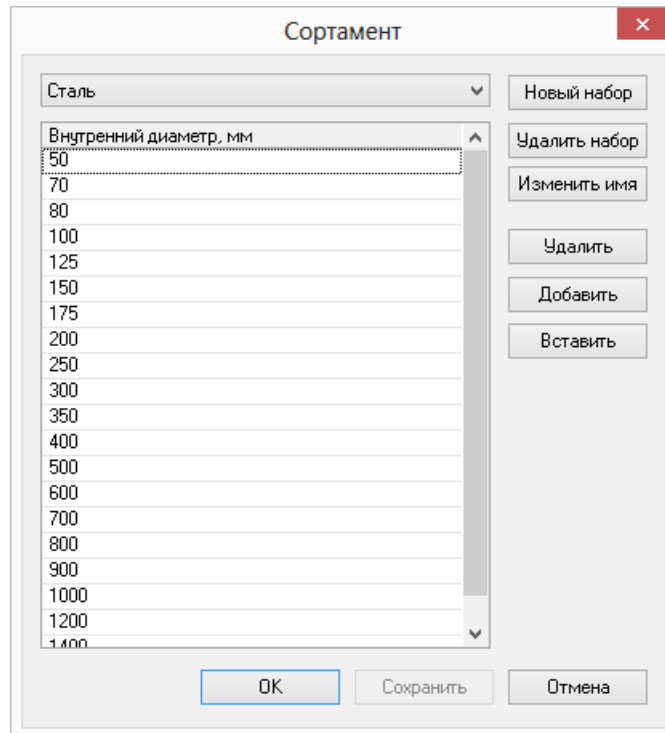
Рисунок 20.3. Окно «Сортамент»
