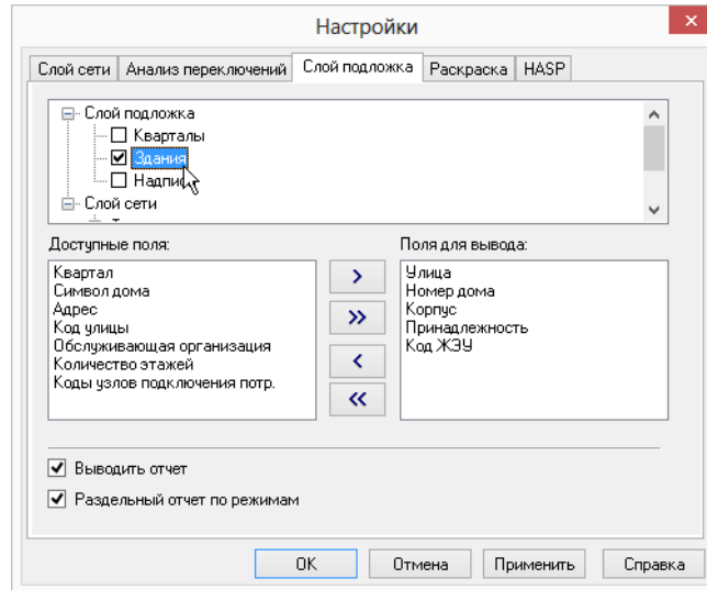
Рисунок 16.12. Настройка слоя-подложки
