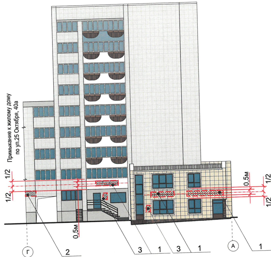
Боковой фасад
