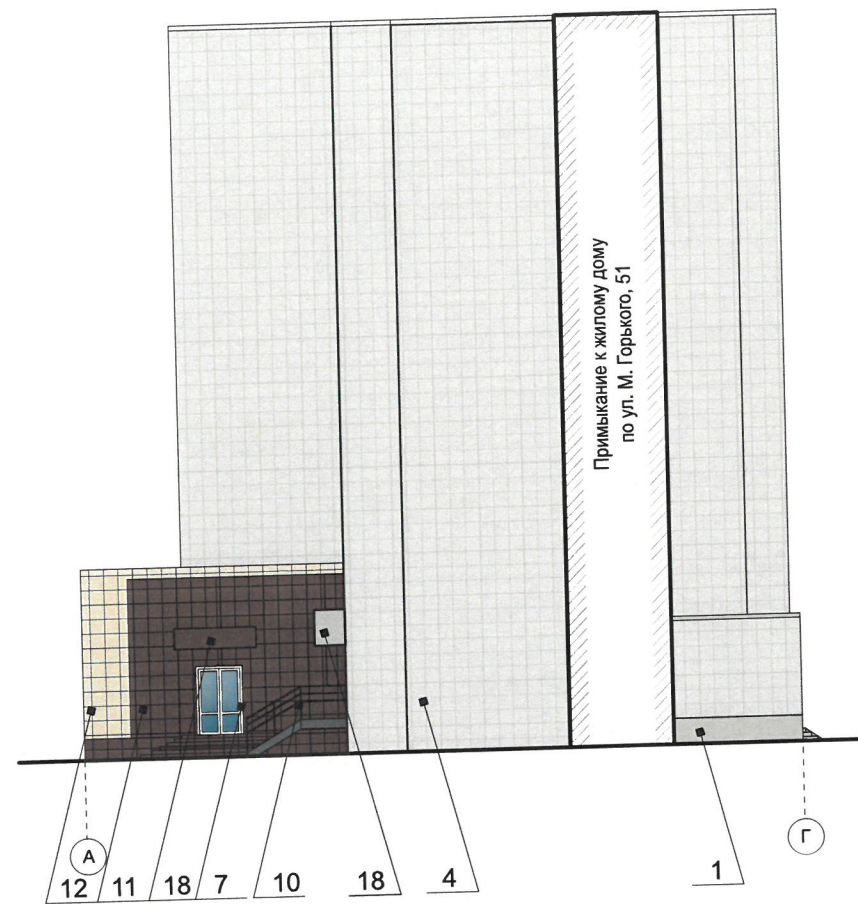
Боковой фасад
