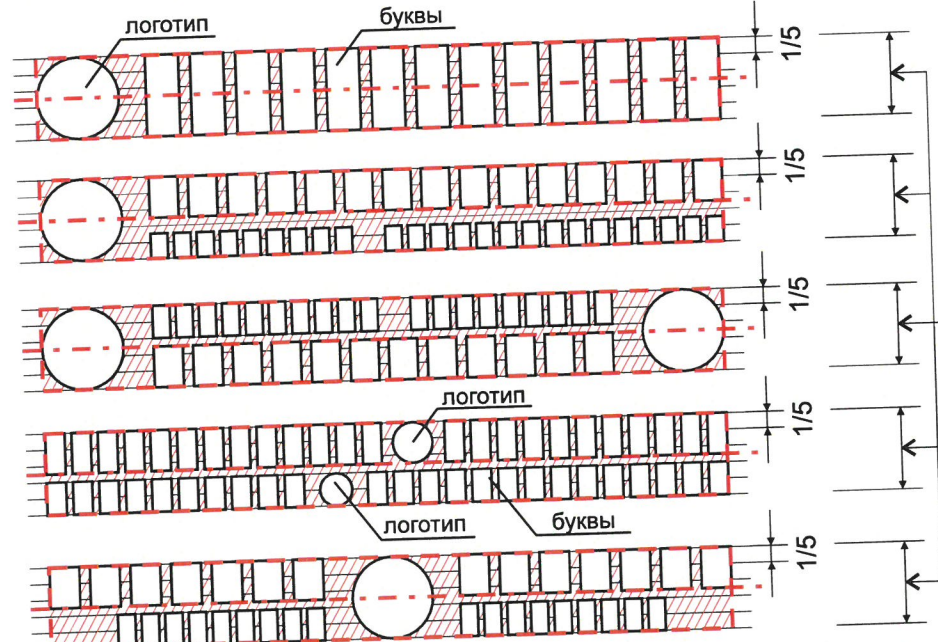
Схема компоновки объемных букв и/или логотипов
