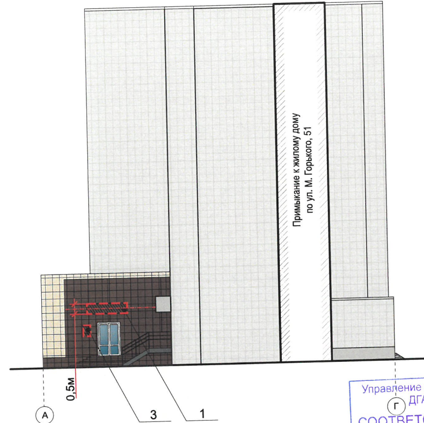
Боковой фасад
