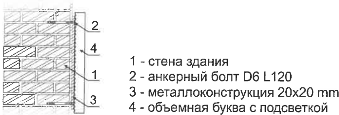
Узел крепления вывески поз. 2
