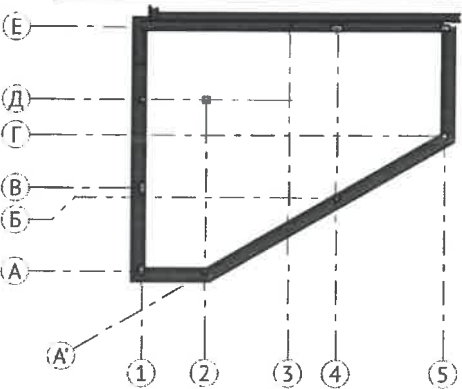
План координационных осей здания
