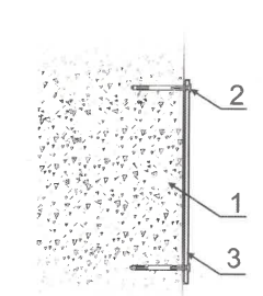
Узел крепления вывески поз. 1
