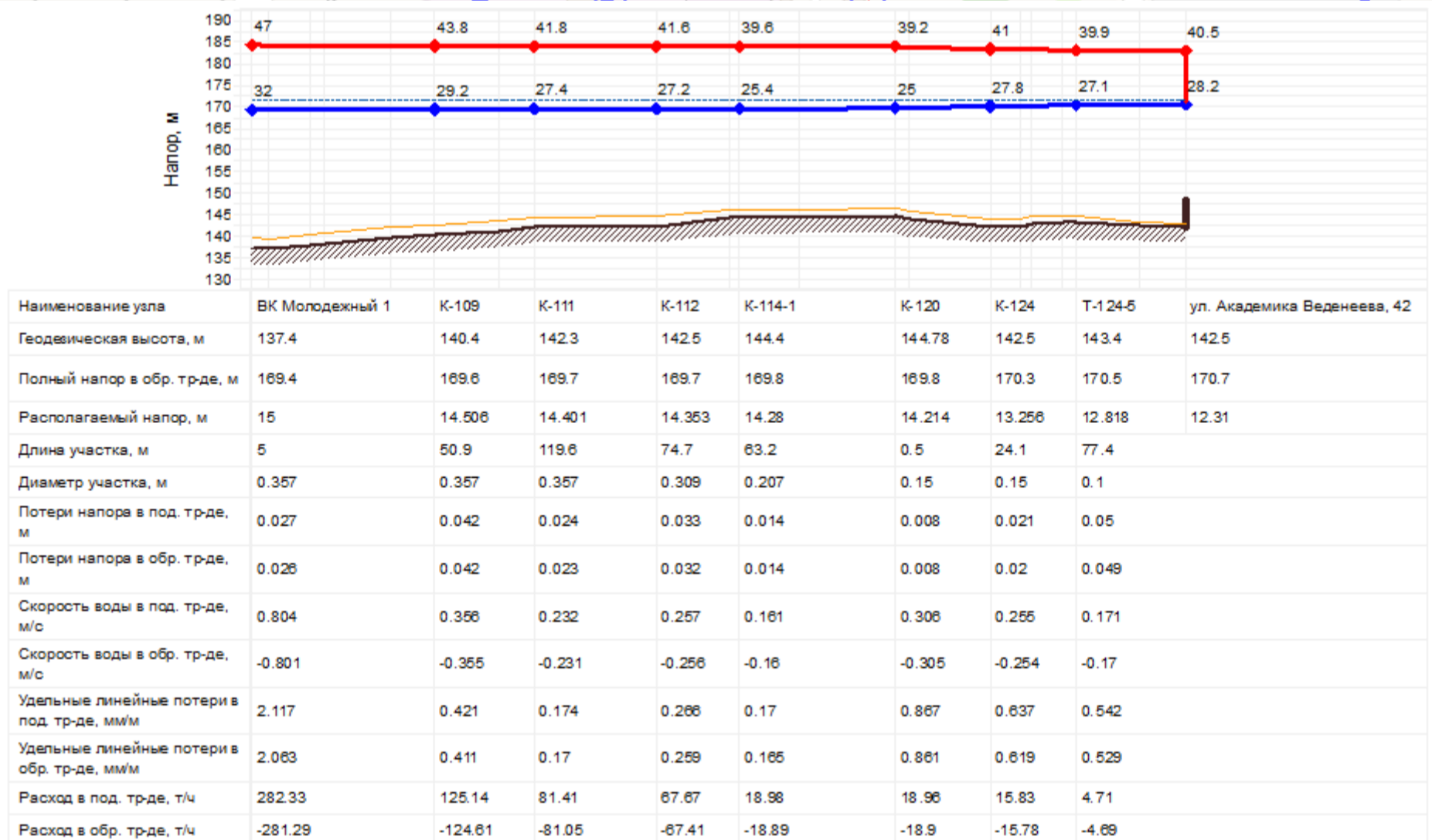
Рисунок 20 – Перспективный пьезометрический график ВК Молодежная – ул. Академика Веденева, 42
