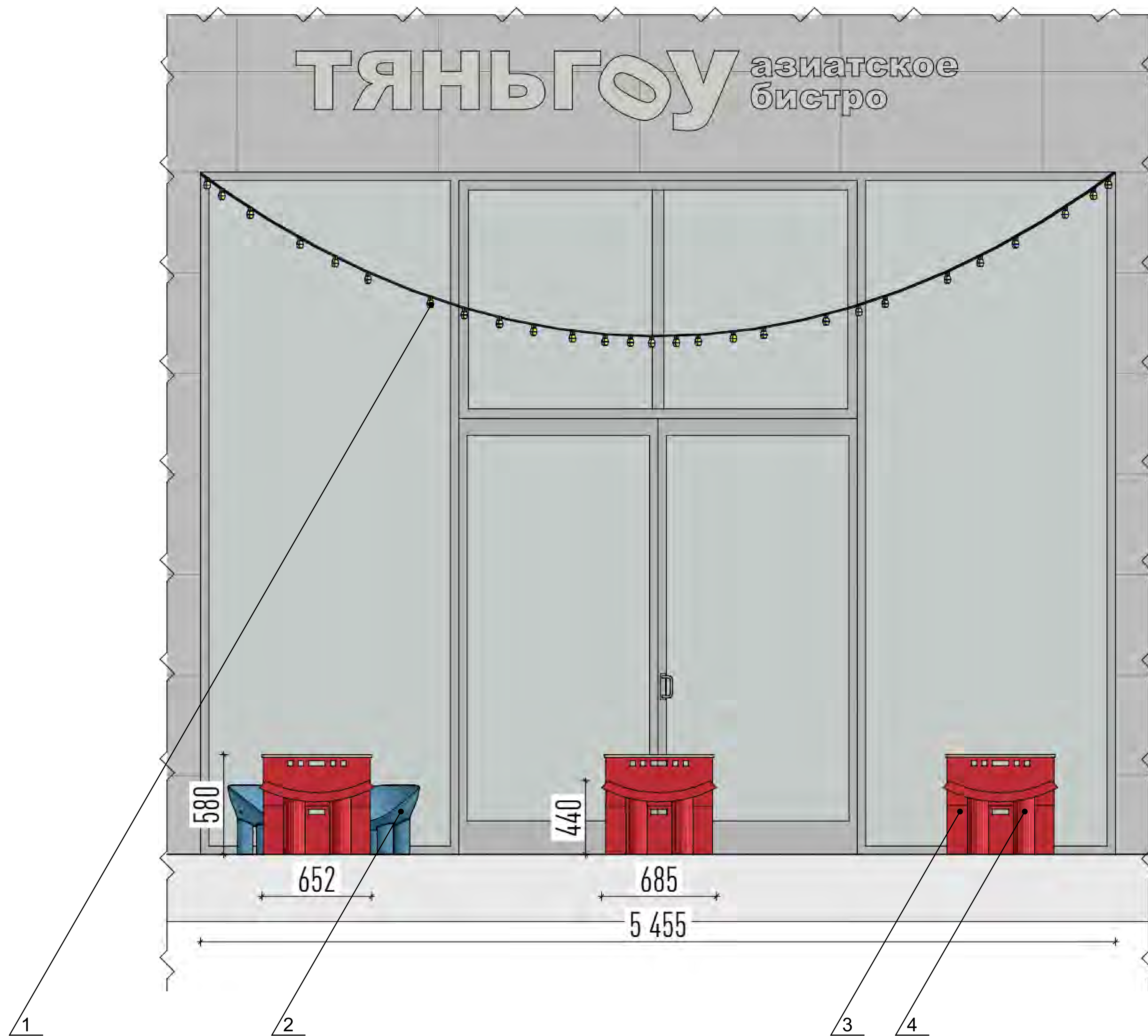
Вид спереди 1:30 (северный фасад)
