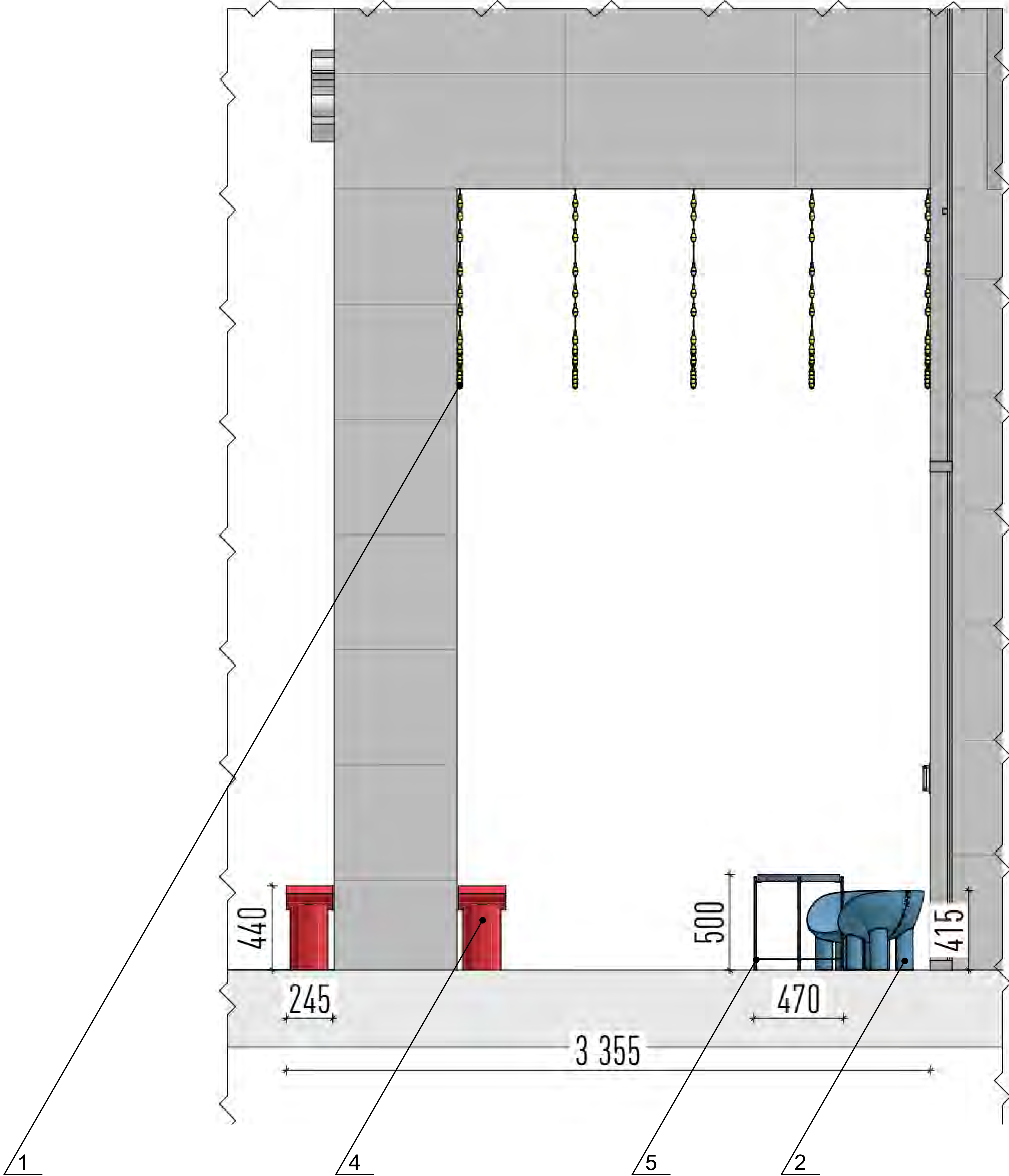
Вид спереди 1:30 (западный фасад)
