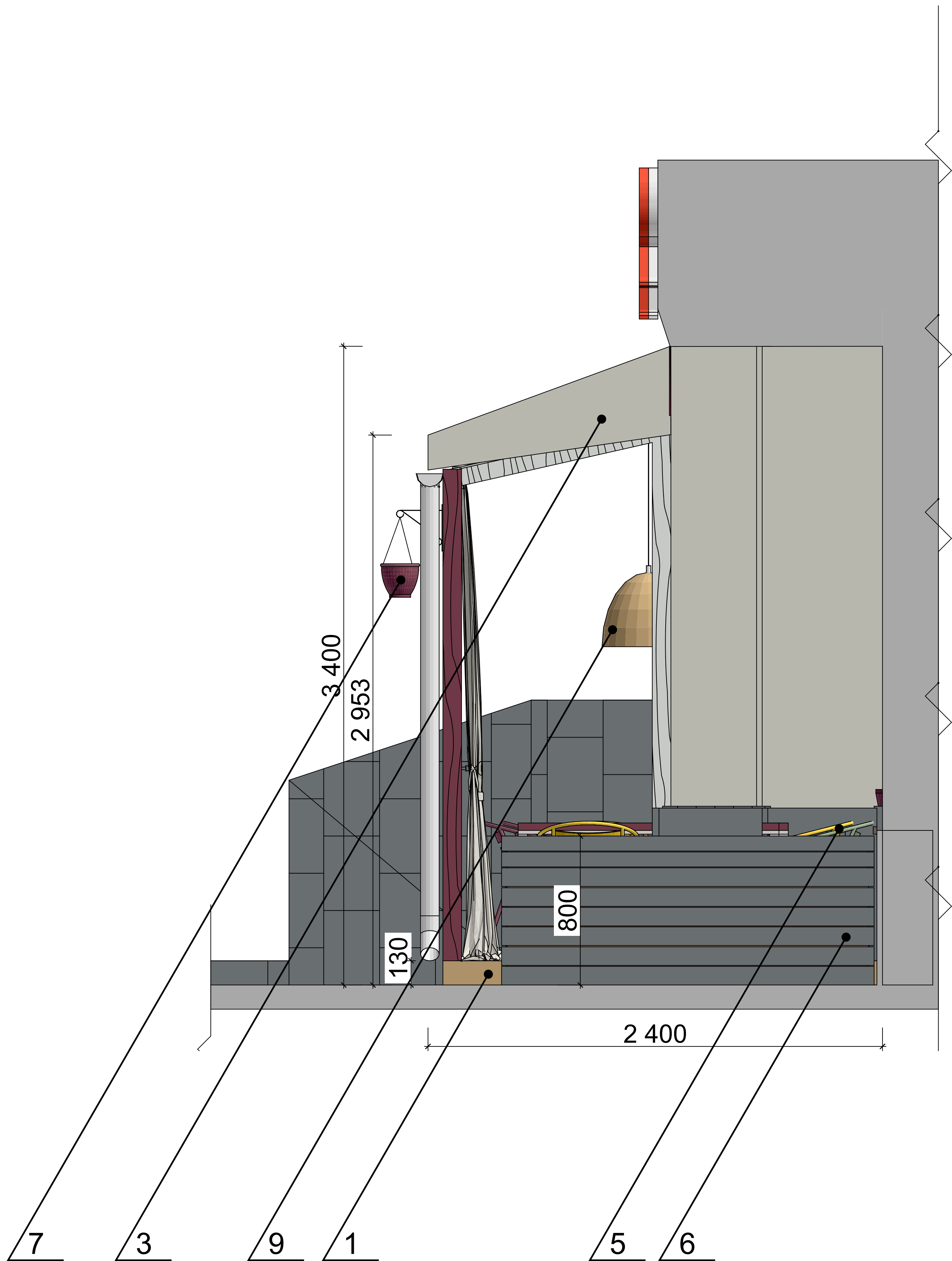
Вид сбоку 1:50 (южный фасад)
