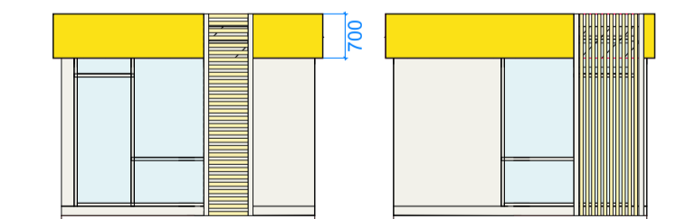
боковые фасады
