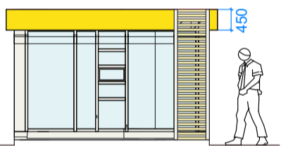
главный фасад
