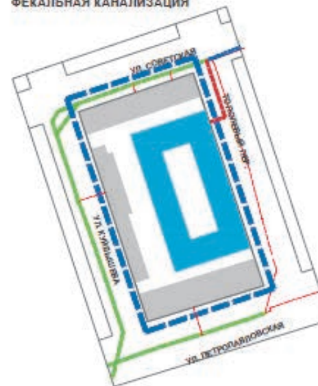
ФЕКАЛЬНАЯ КАНАЛИЗАЦИЯ
