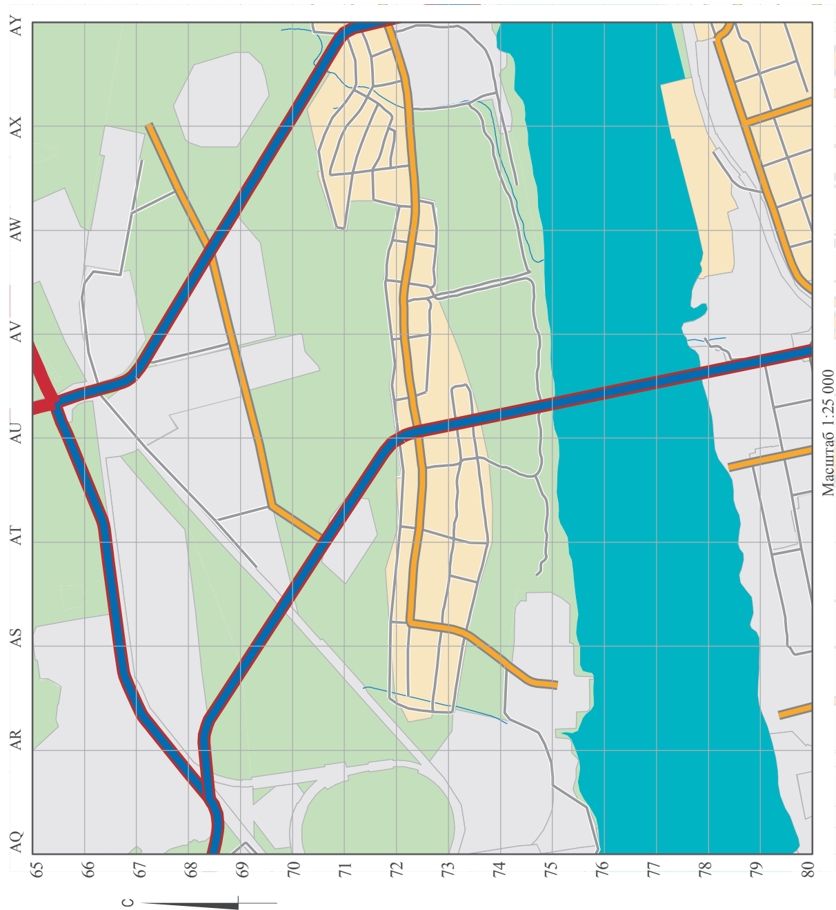
Фрагмент Карты 2.1.1. Виды улиц и дорог по назначению
