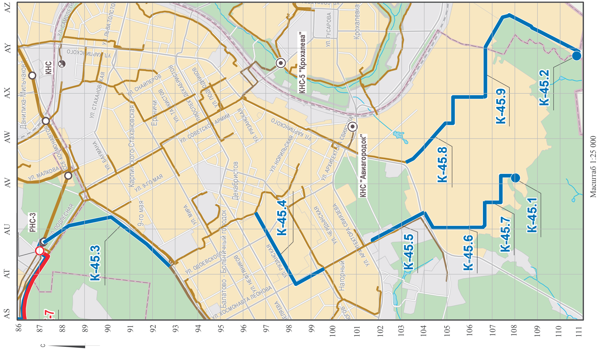
Фрагмент Карты 2.2.2. Развитие сети объектов водоотведения
