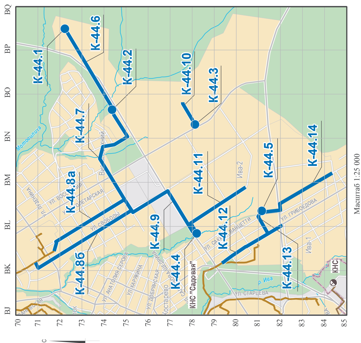
Фрагмент Карты 2.2.2. Развитие сети объектов водоотведения
