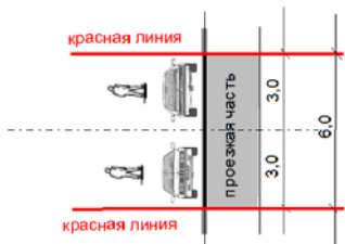
Профиль квартальной улицы в границах проектирования
