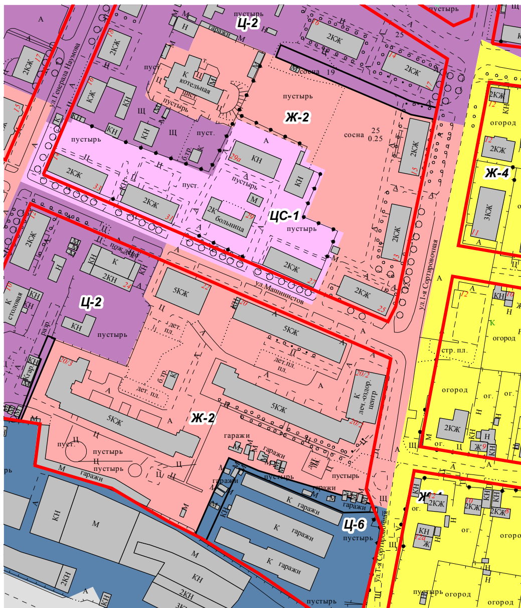
Рисунок 4. Схема предложения в части изменения карты градостроительного зонирования города Перми Правил для территории квартала, ограниченного ул. Генерала Наумова, ул. Машинистов, ул. Сортировочной 1-й и квартала, ограниченного ул. Генерала Наумова, ул. Машинистов, ул. Сортировочной 1-й и ул. Ветлужской
