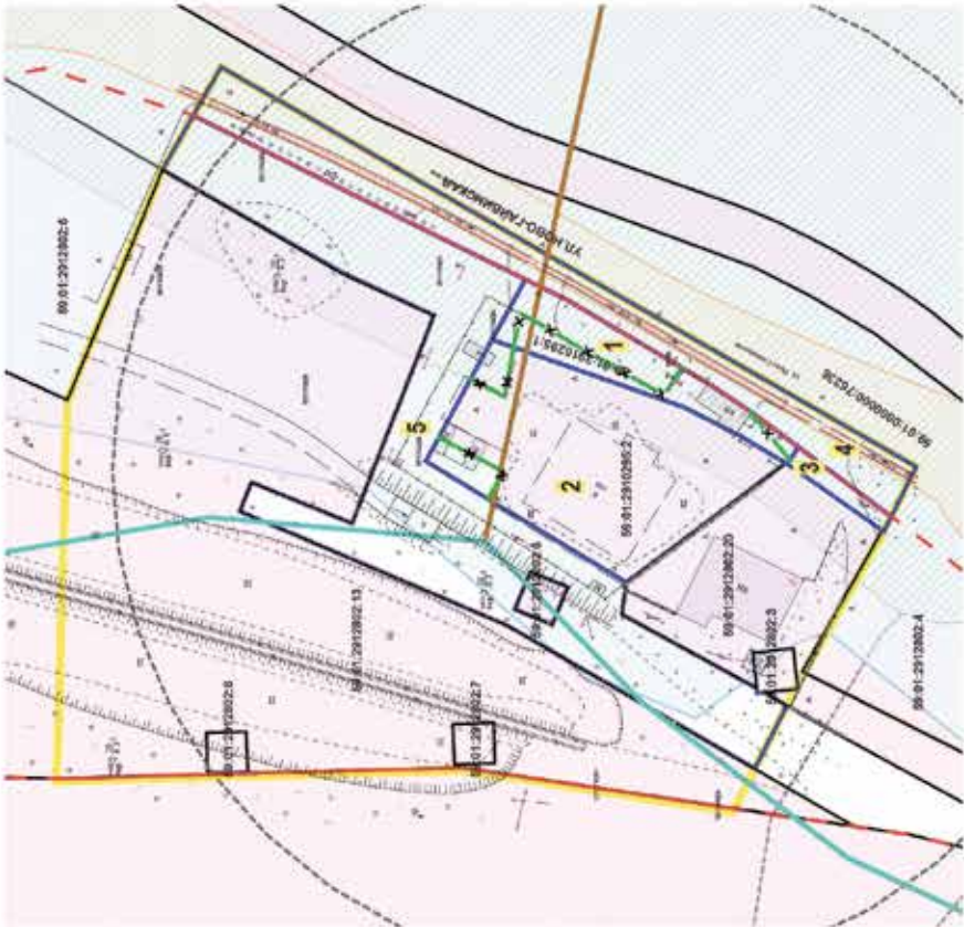
Чертеж межевания территории
