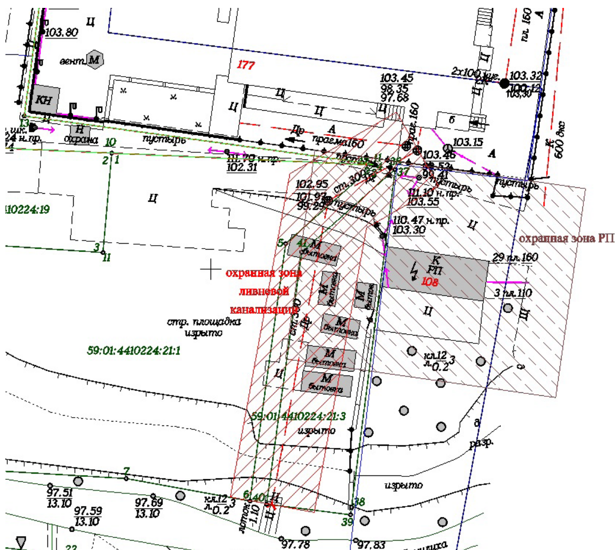
Рисунок. 1. Расположение охранных зон ливневой канализации и РП
