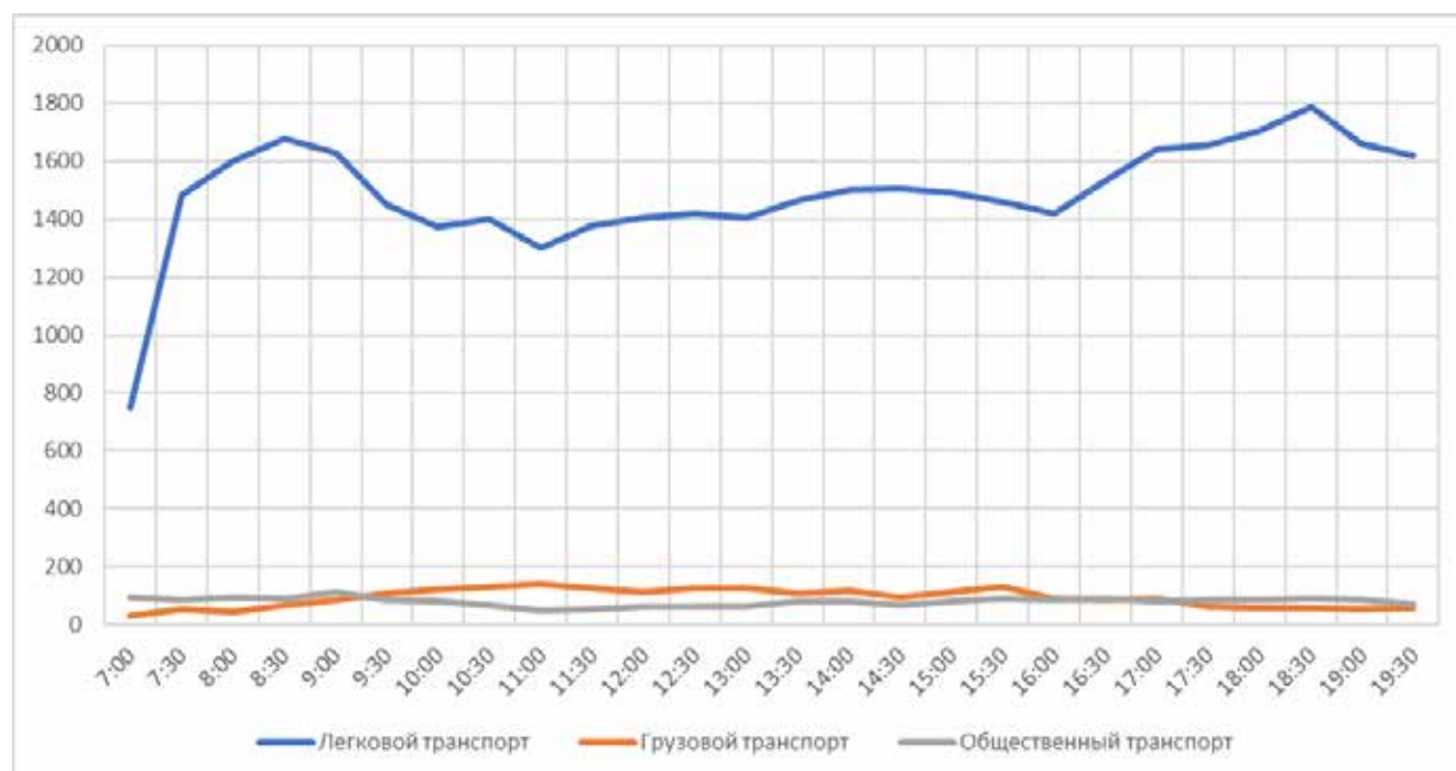
График дневных колебаний интенсивности транспортных потоков в городе Перми, авт./30 мин.
