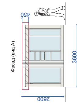
Главный фасад
