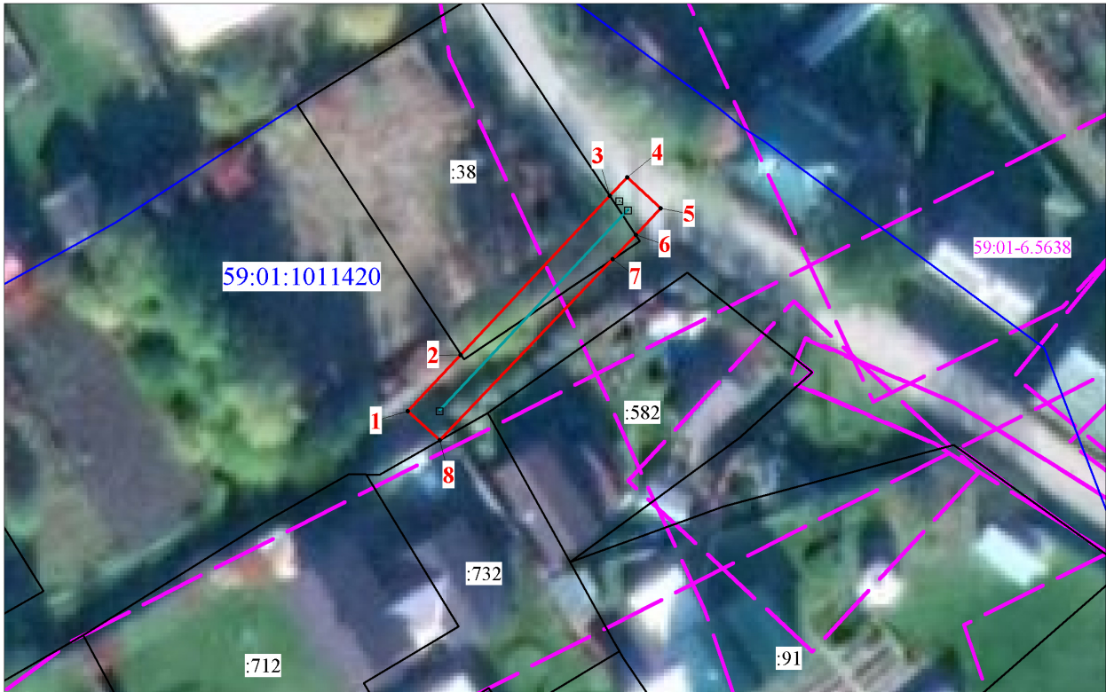
Масштаб 1:500
